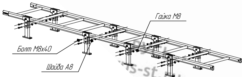
2. Крепление кровельного кр-на.
