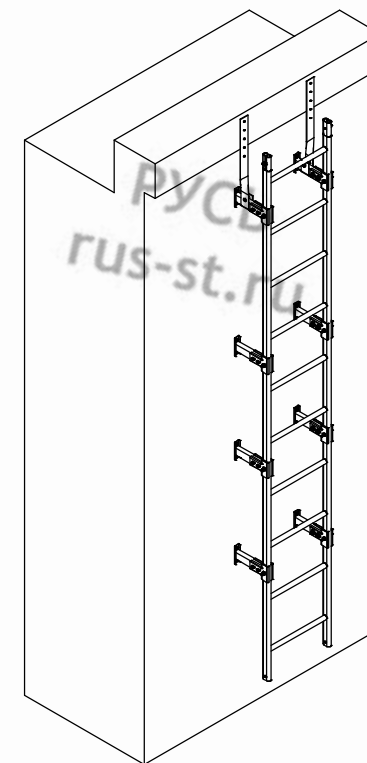
4. Итоговый вид смонтированной лестницы.
