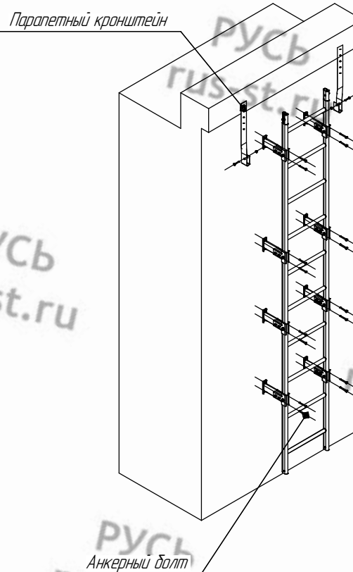
3. Крепление кронштейнов к лестнице. Монтаж готовой лестницы к фасаду.
