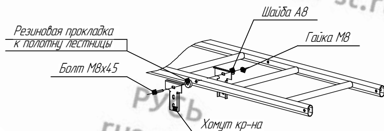
1. Крепление хомута кр-на к лестнице.
